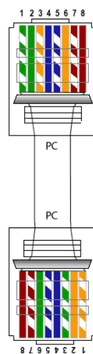
Kabel typu Crossover
